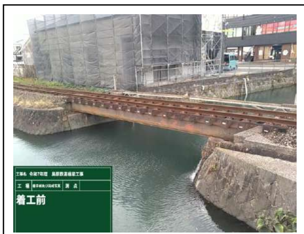
島原駅～霊丘公園体育館駅間 音無川 橋桁交換及び重防食塗装（施工前）
