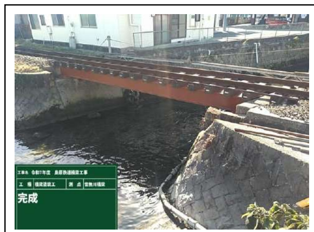
島原駅～霊丘公園体育館駅間 音無川 橋桁交換及び重防食塗装（施工後）
